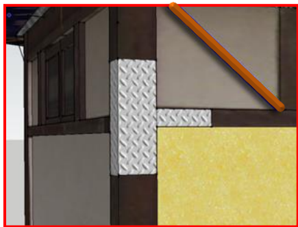
테두리강판 설치
