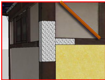
테두리강판 설치
