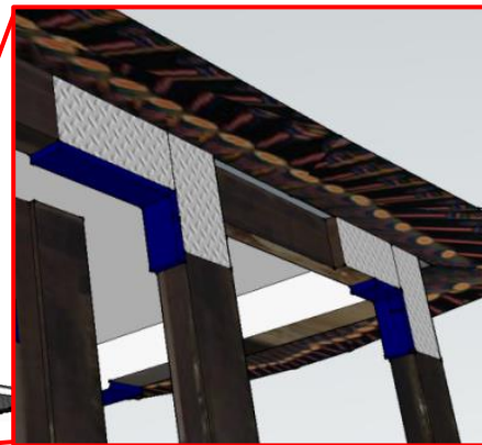
연결부 보강
